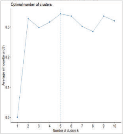
Gambar 1. Jumlah Kluster Optimal
